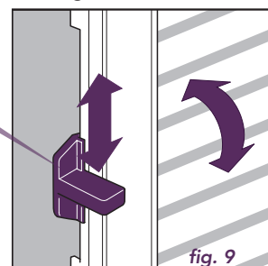
Poignée d'inclinaison
